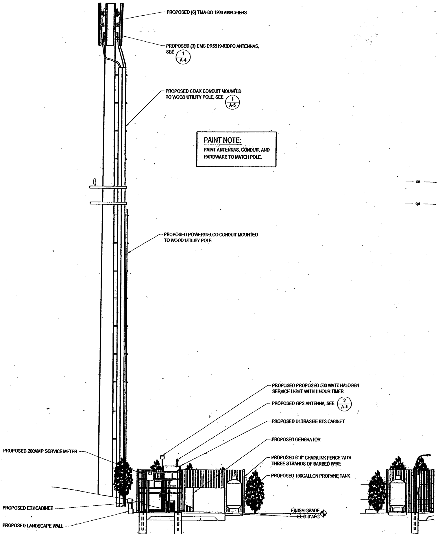
SOUTH ELEVATION 22x34 SCALE: 1/4"=1'-0" 11x17 SCALE: 1/8"=1'-0"
